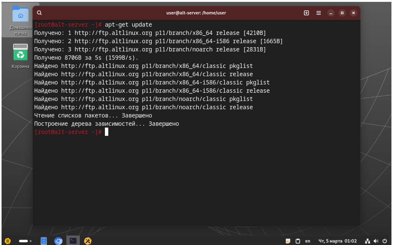
Рис. 2.37. Подготовка пакетного менеджера apt-get
