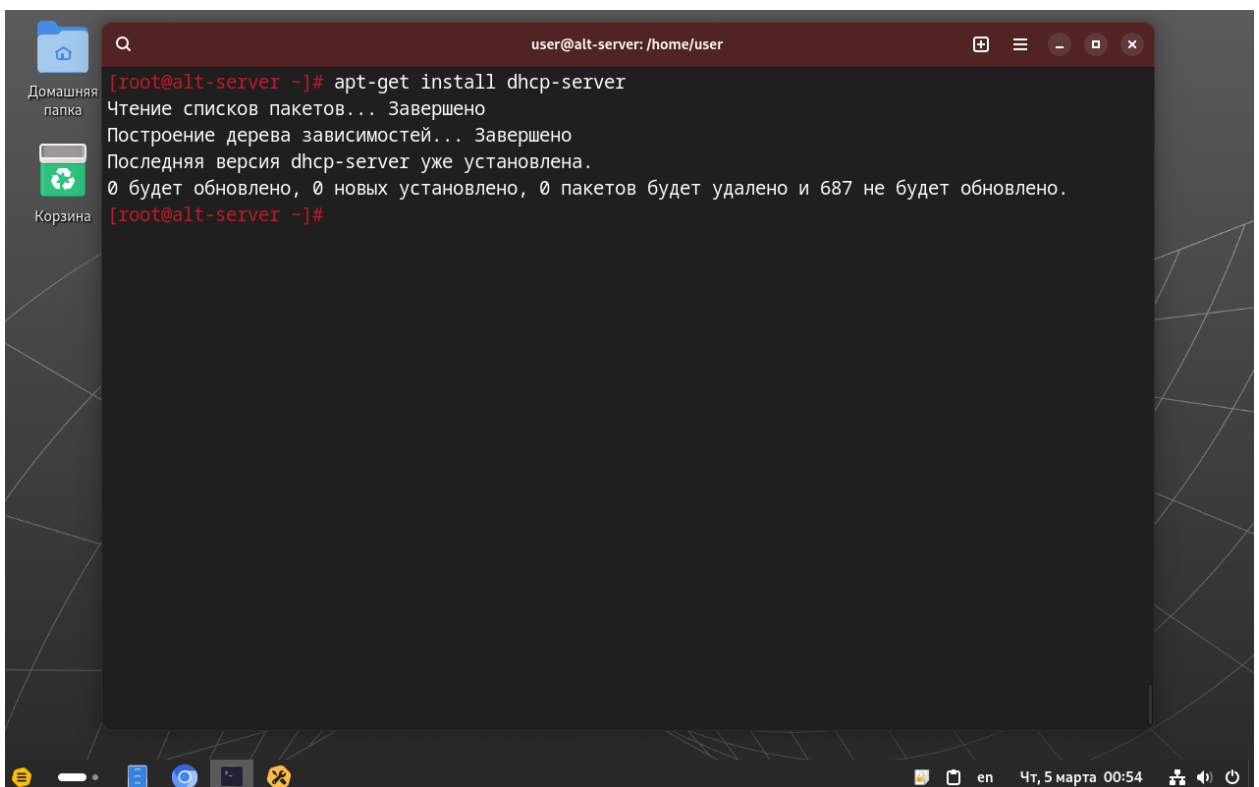
Рис. 2.38. Установка сервера динамических адресов
