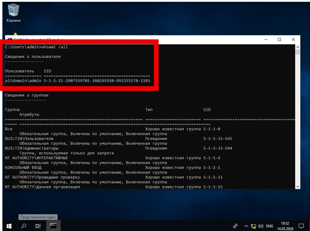
Рис. 4.16. Проверка данных пользователя
