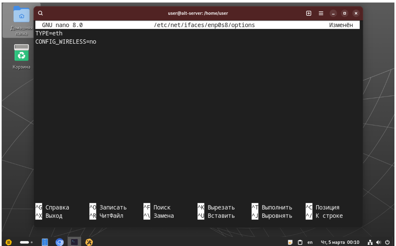
Рис. 2.10. Конфигурационный файл сетевого интерфейса до редактирования Приведем данный файл к следующему виду рис. 2.11.
