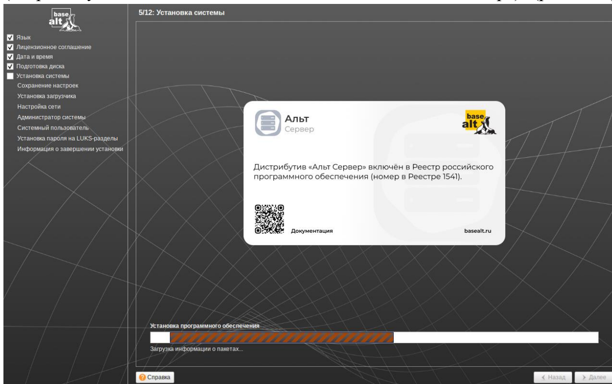
Рис. 1.25. Установка системы
