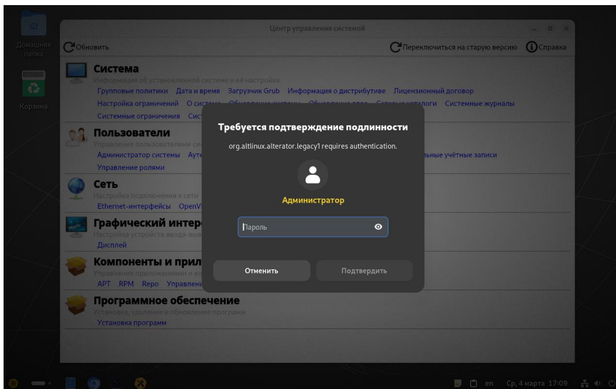
Рис. 2.2. Проверка подлинности
