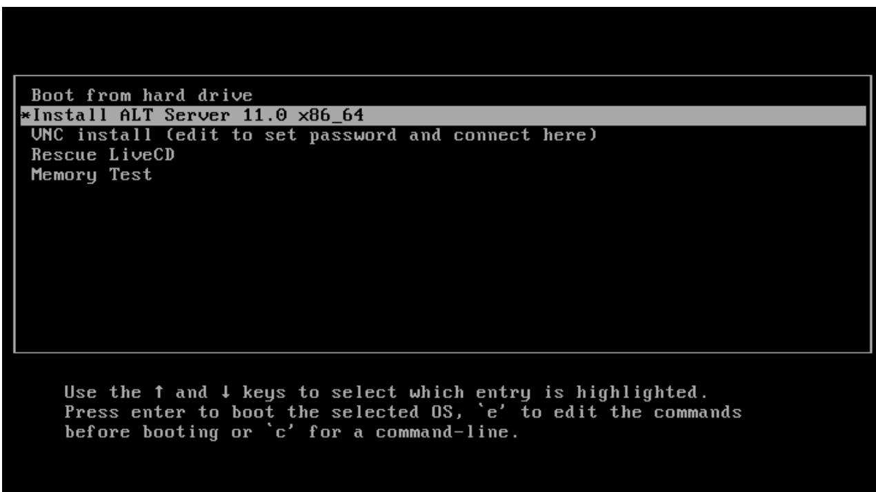
Рис 1.12. Загрузочное меню
