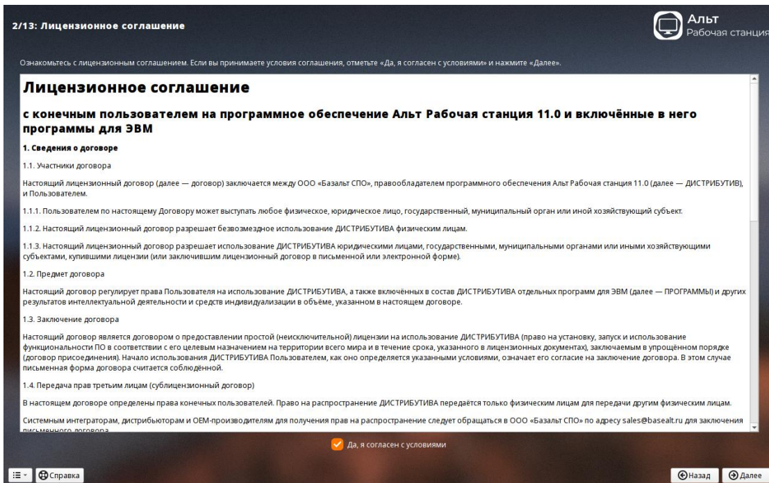
Рис. 3.28. Лицензионное соглашение
