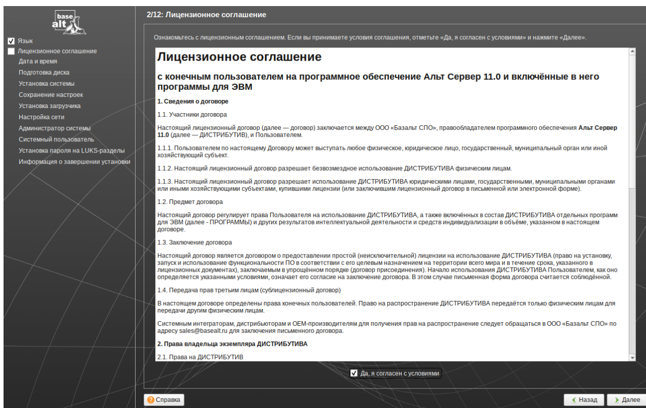
рис.1.15. Лицензионное соглашение
