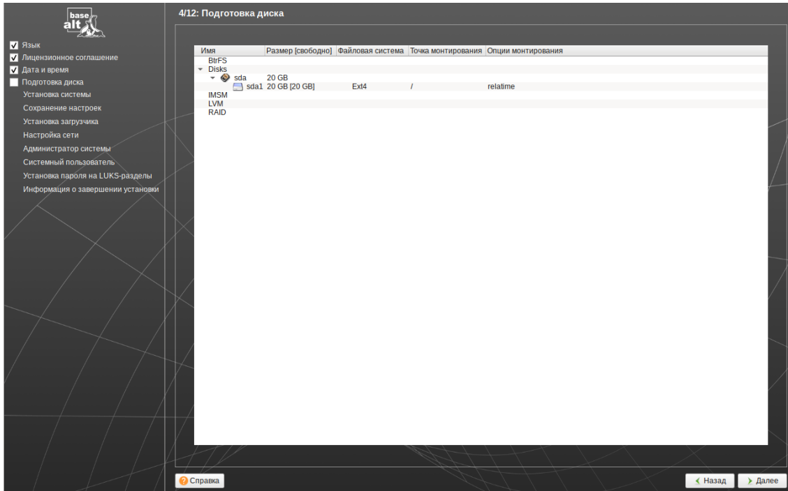
Рис. 1.22. Подготовка диска
