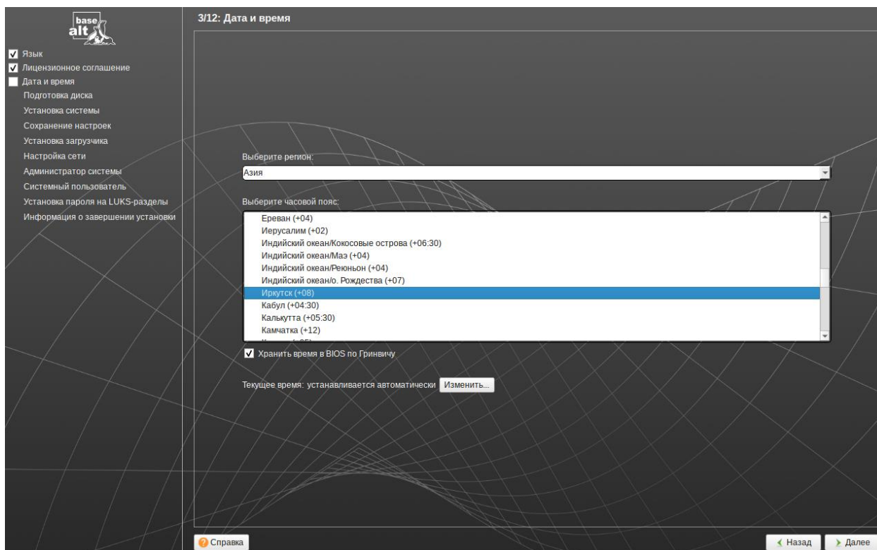
Рис. 1.16. Часовой пояс
