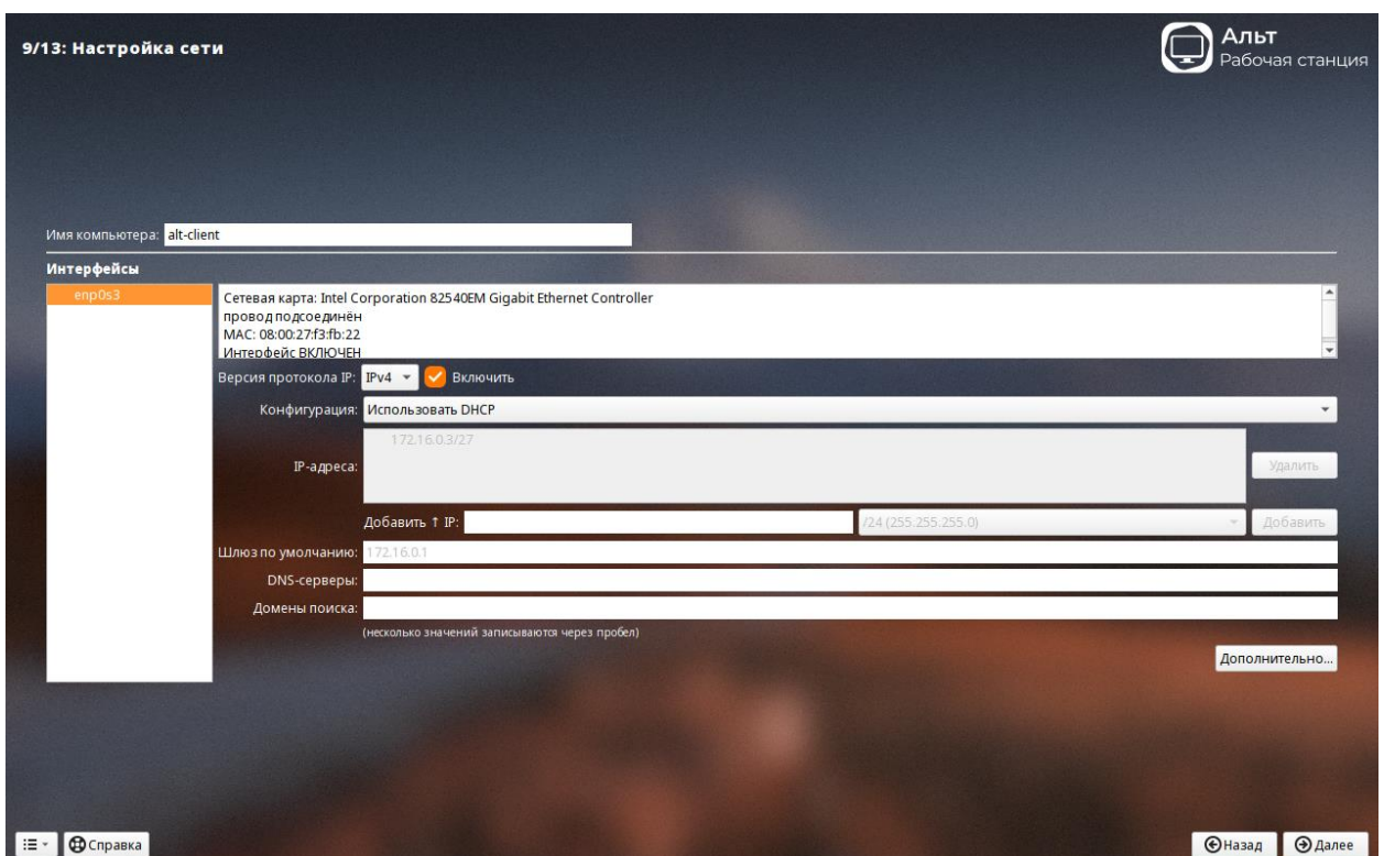
Рис. 3.36. Назначение сетевых параметров и имени хоста
