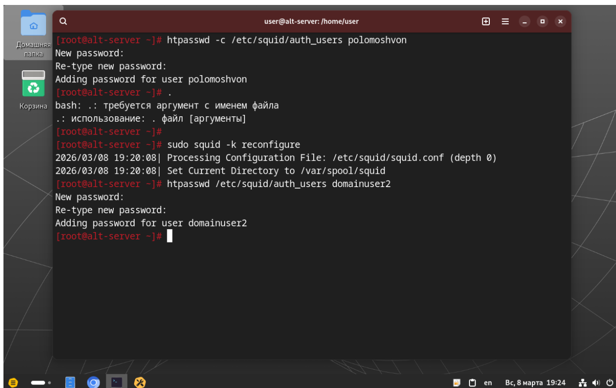
Рис. 2.36. Создание пользователей для прокси сервера
