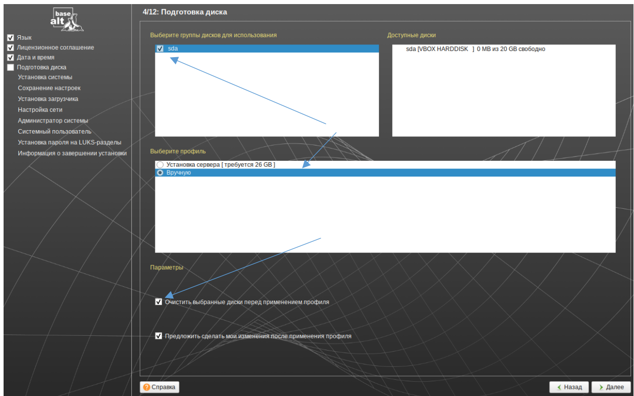
Рис. 1.17. Выбор диска для установки
