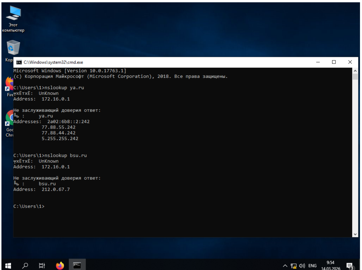
Рис. 4.7. Проверка работы dns сервера
