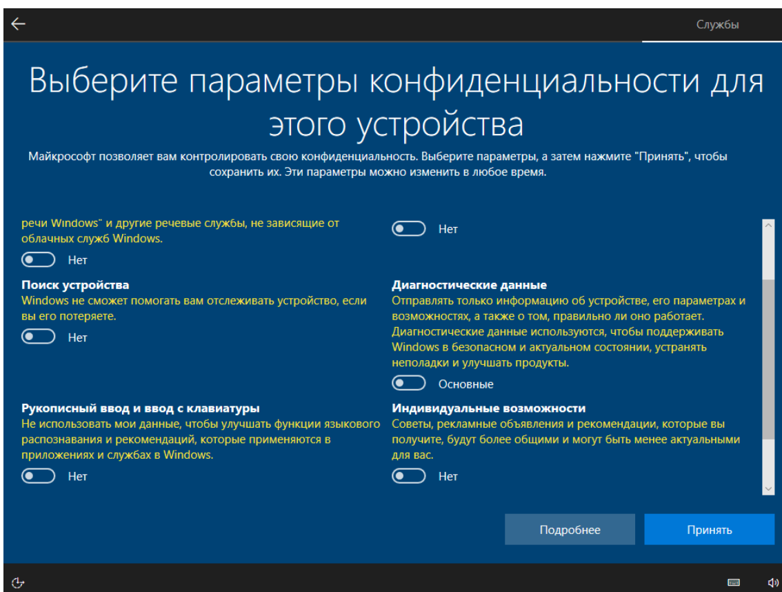
Рис. 3.21. Параметры конфиденциальности
