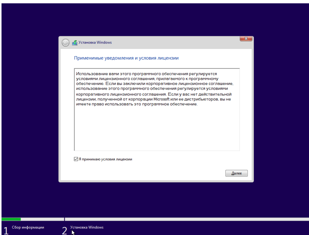
Рис. 3.9. Лицензионное соглашение
