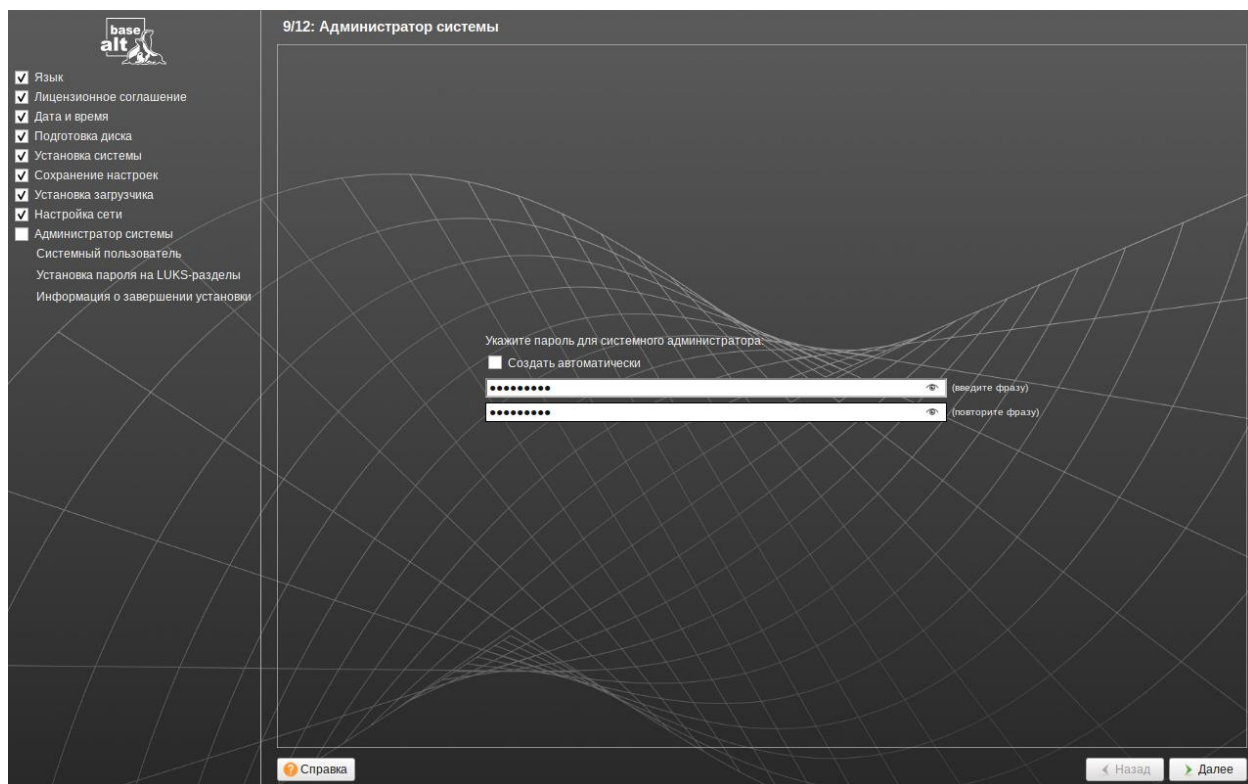
Рис. 1.28. Пароль суперпользователя
