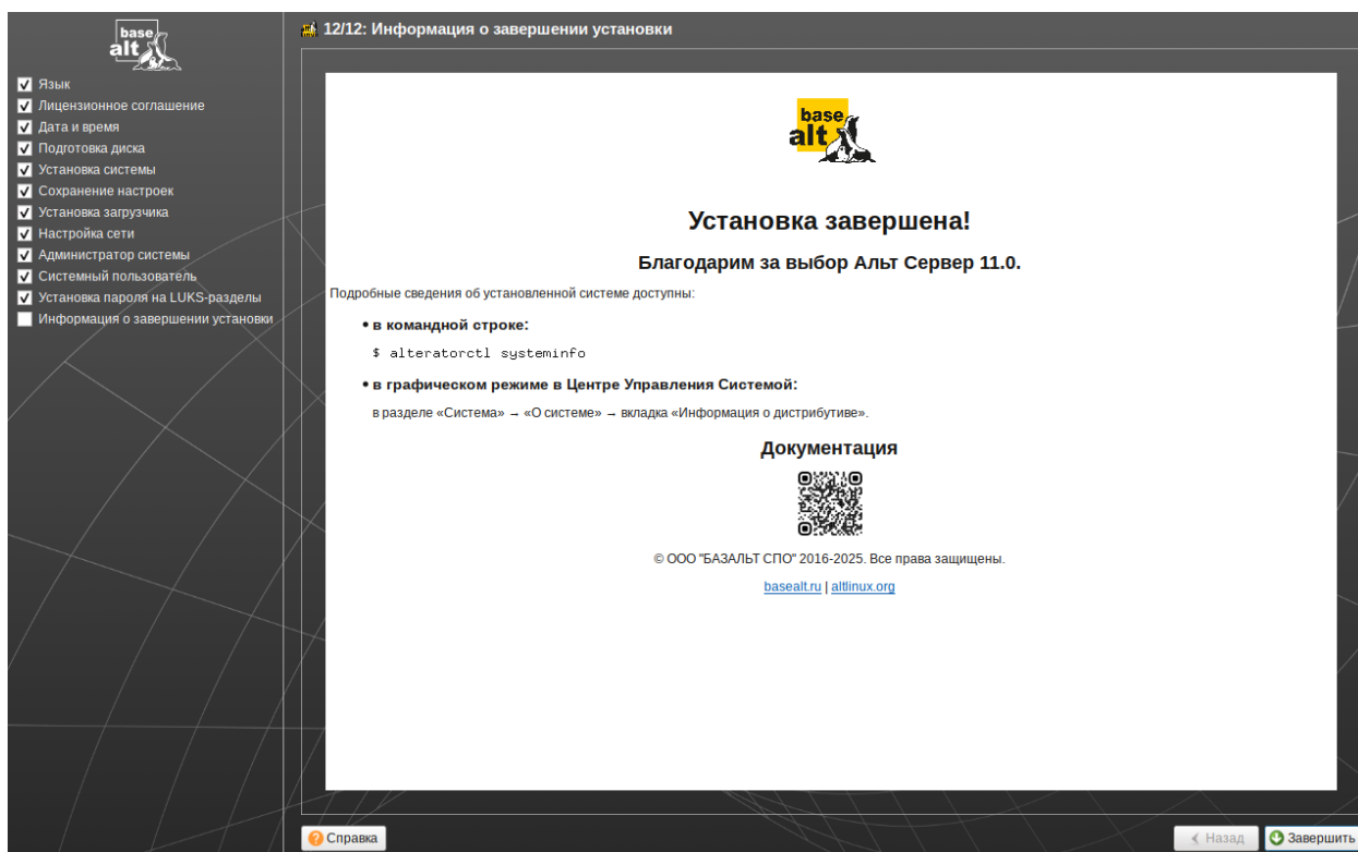
Рис. 1.30. Завершение установки
