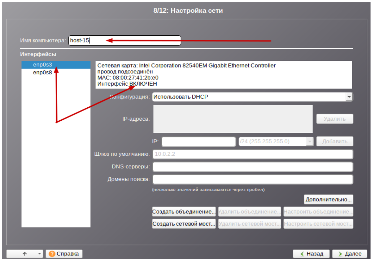
Рис. 1.27. Настройка имени хоста и сетевых настроек
