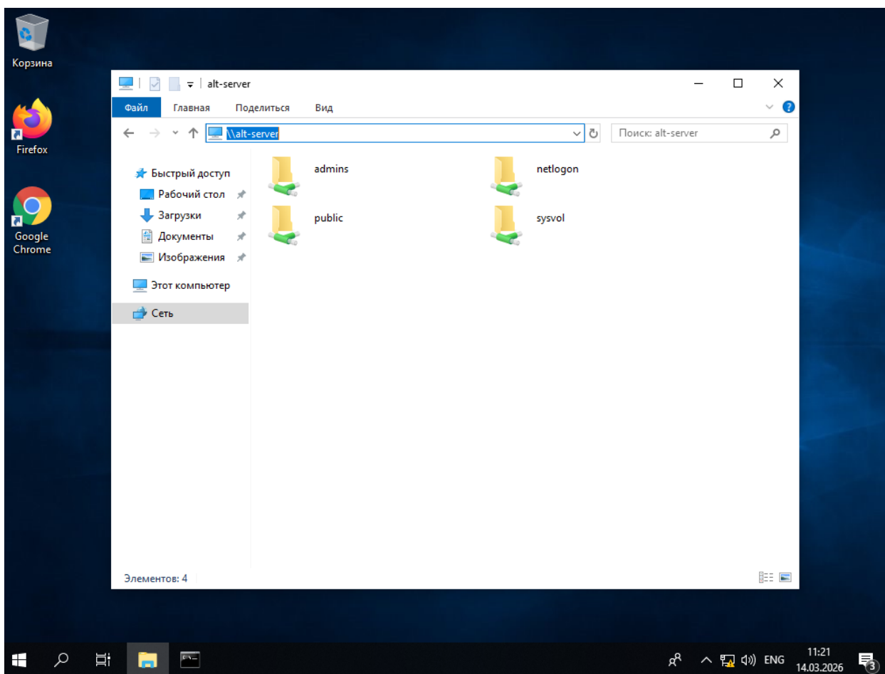
Рис. 4.20. Подключение к файловому серверу с использованием проводника
