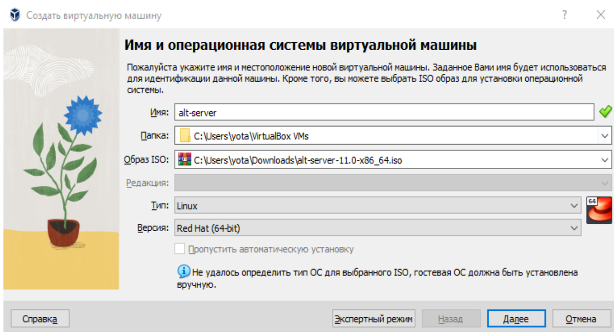
Рис. 1.2. Создание новой виртуальной машины
