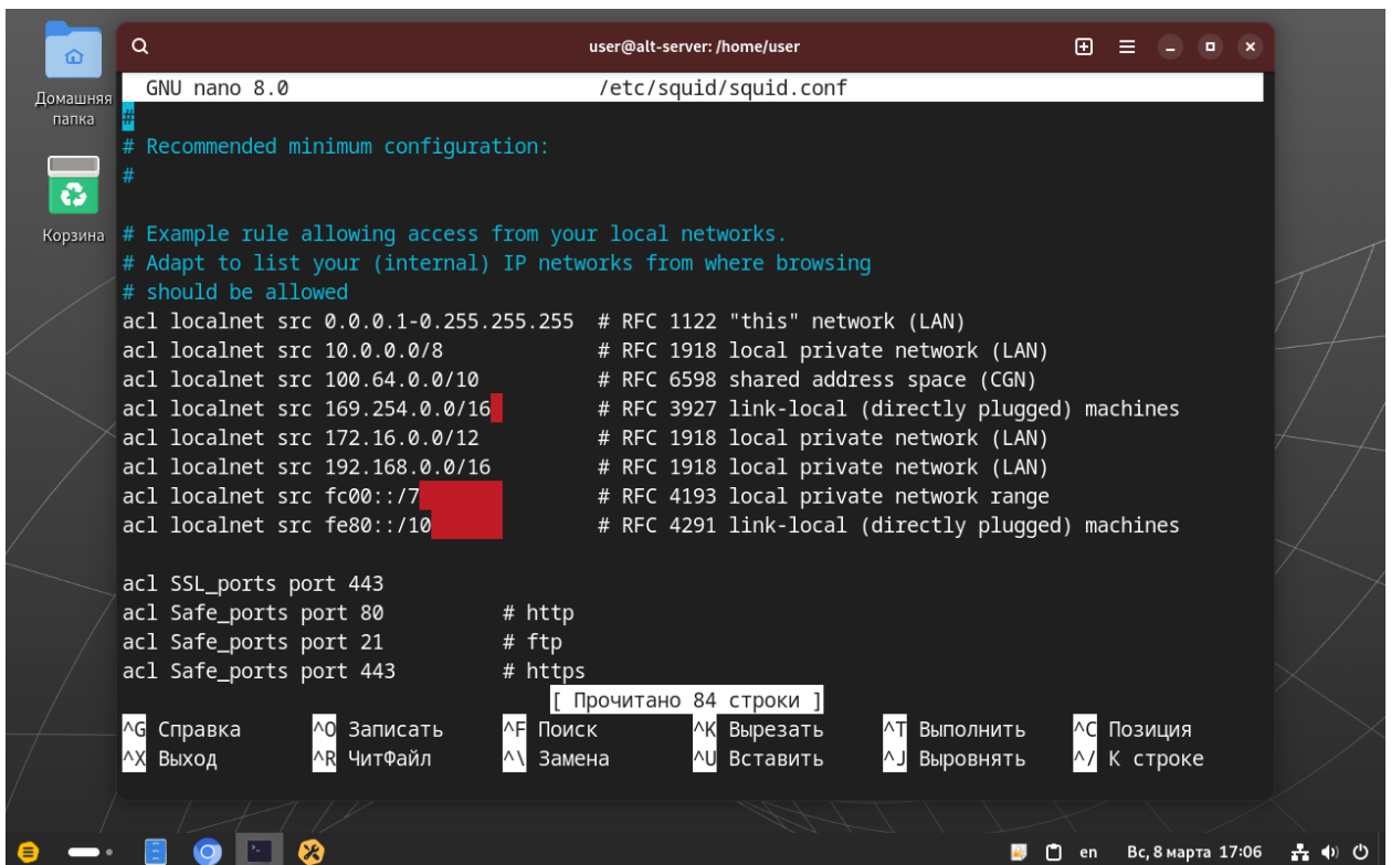
Рис. 2.32. Вид файла конфигурации прокси-сервера Squid по умолчанию
